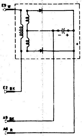
FIG. H TP152950 RECTIFIER ASSEMBLY
